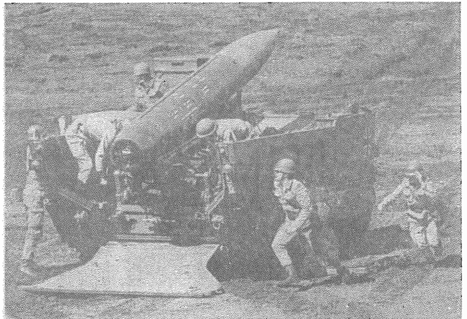
نمونه از موشک کوتاه برد "لاناس" که آمریکایی‌ها می‌خواهند مدرنیزه کنند
