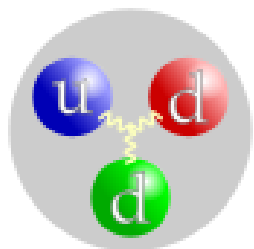
تصویر ۳: ساختار کوانتومی نوترون ۱
